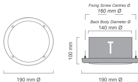
Reflex Recess 190 - Mini 190mm Ø
